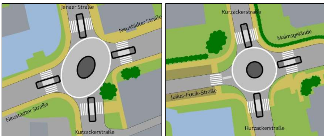
Abb. 49 Prinzipskizzen Umgestaltung zum Minikreisverkehr
