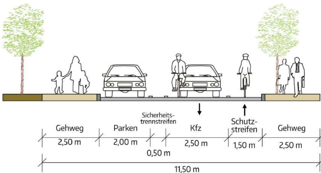
Abb. 39 Vorschlag Querschnittsaufteilung Ernst-Thälmann-Straße
